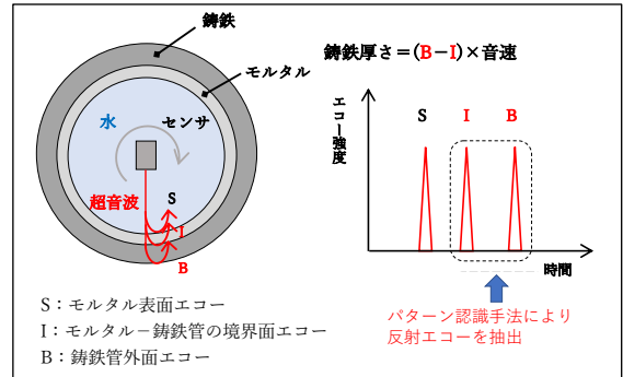
図1 測定原理
