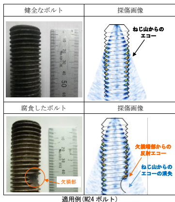
適用例 (M24 ボルト)
