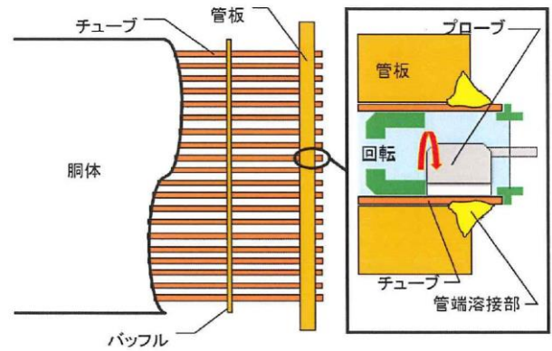
図1 管端溶接部検査イメージ
