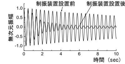
図10 制振装置による減衰性の向上
