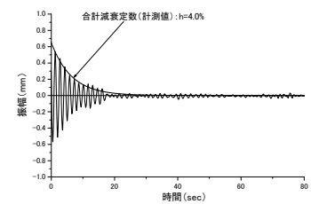
(b) 装置設置後
